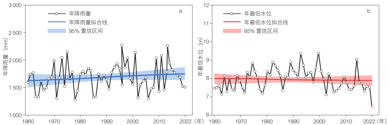
图4 鄱阳湖流域1960—2022年降雨量(a)和年最低水位(b)变化情况
