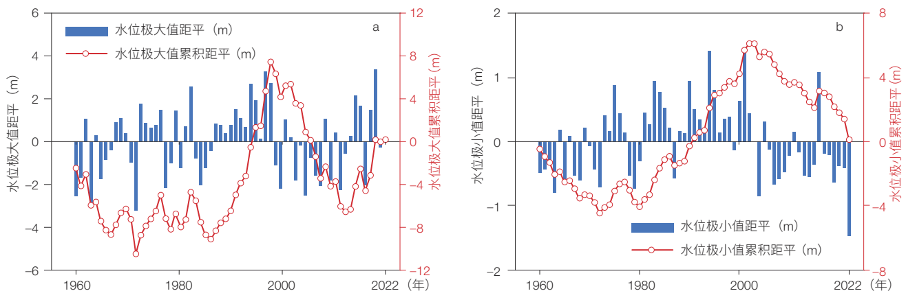
图 3 1960—2022 年鄱阳湖水水位极大值 (a) 和极小值 (b) 距平和累积距平
