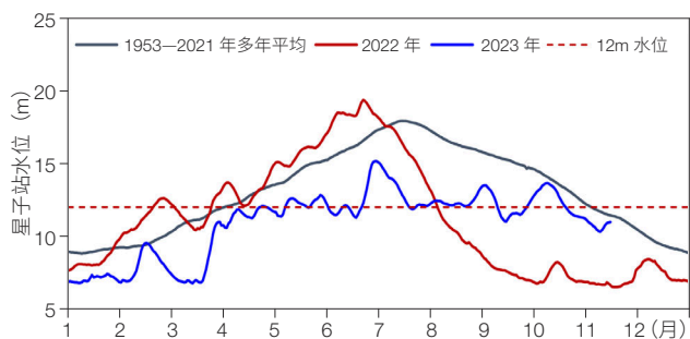
图2 鄱阳湖2022、2023年水位与多年（1953—2021年）平均值对比
