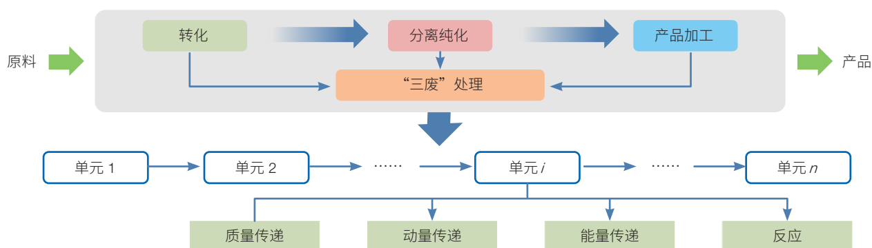
图4 工业过程单元强化示意图
