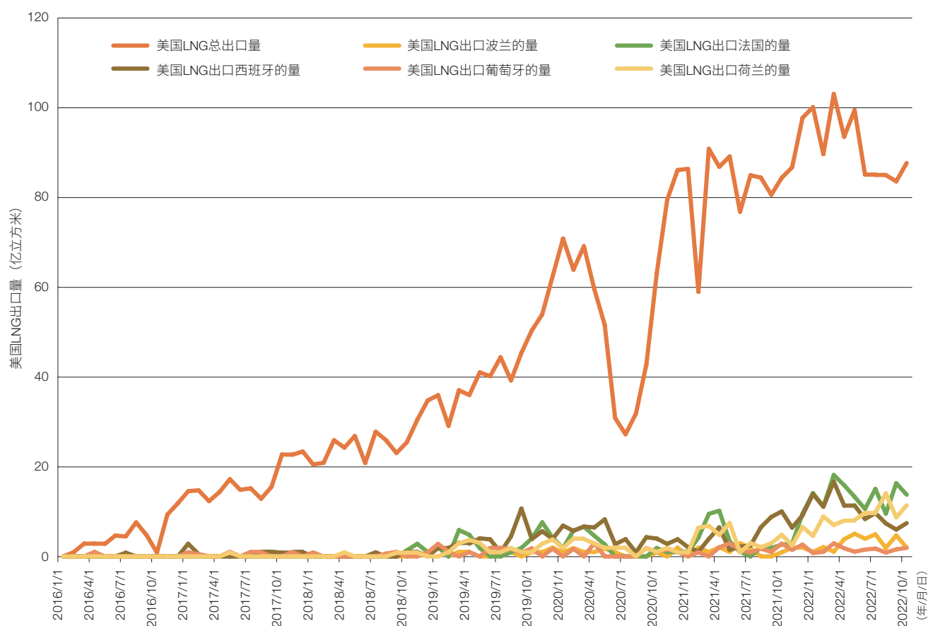
图4 2016年1月—2022年10月美国液化天然气（LNG）总出口量及其出口到部分欧洲国家的情况
