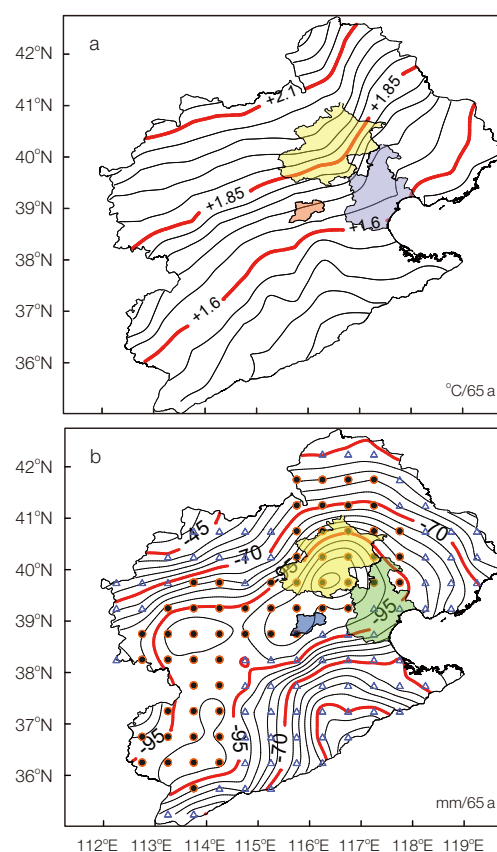
图2 1951—2015年海河流域气温（a）和降水量（b）的线性变化趋势
