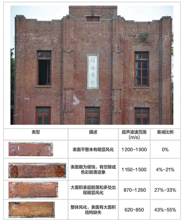
图3 之江大学钟楼立面不同劣化程度的黏土砖与超声波波速之间的关系 图片由周月娥提供
