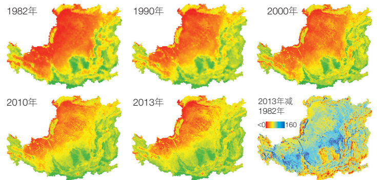
图4 黄土高原植被覆盖度（NDVI）变化时空图谱（1982—2013年）
