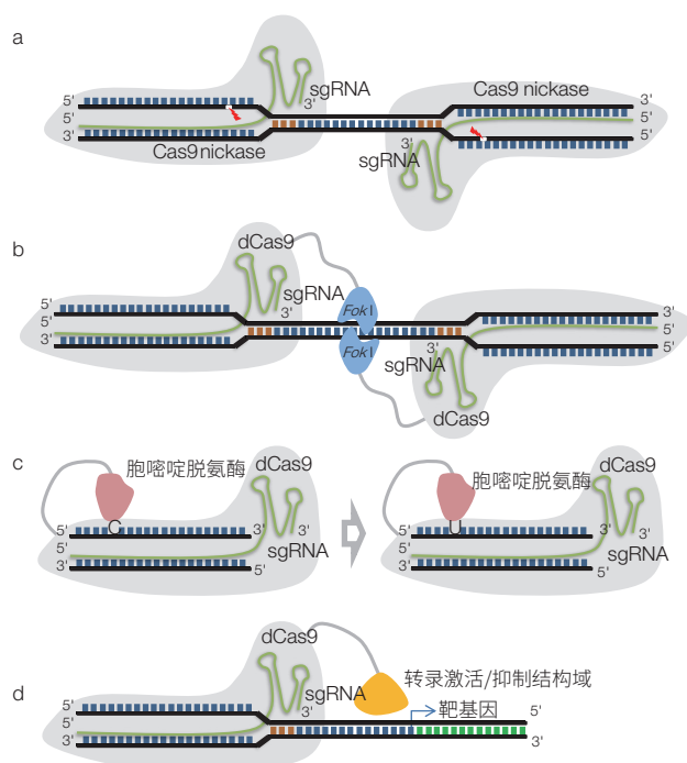
图 2 系列 CRISPR/Cas9 衍生基因编辑技术
