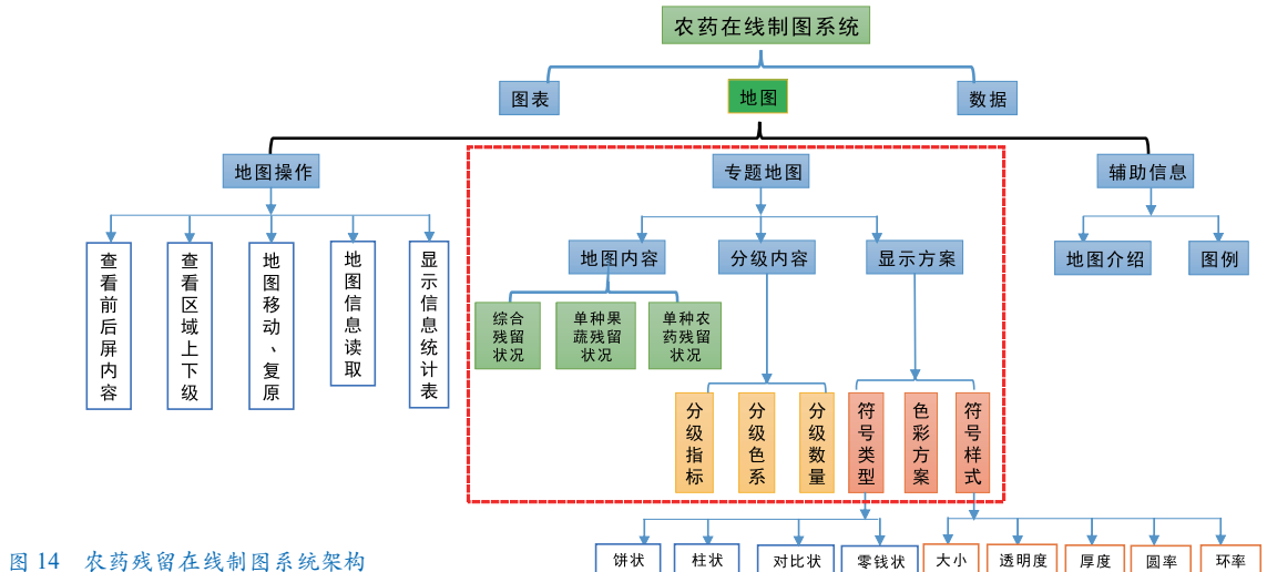
图 14 农药残留在线制图系统架构
