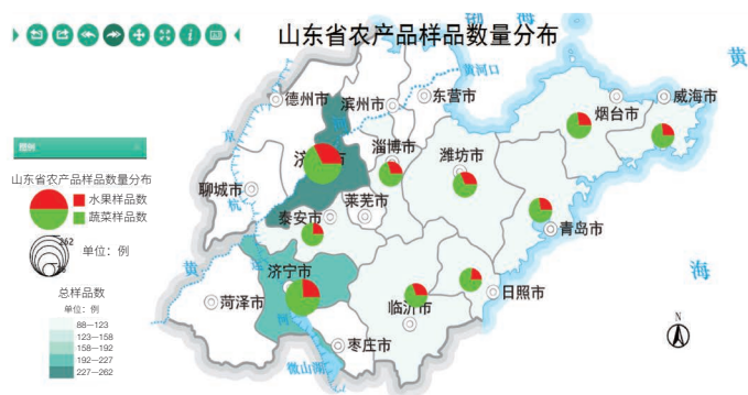
图 15 山东省水果蔬菜样品数量分布图
