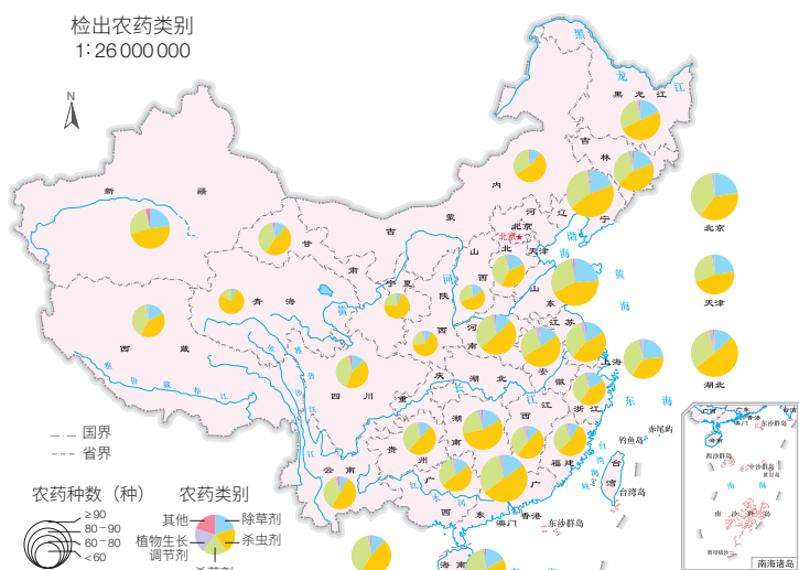
图20 全国31个省/直辖市市售水果蔬菜样品检出农药类别
