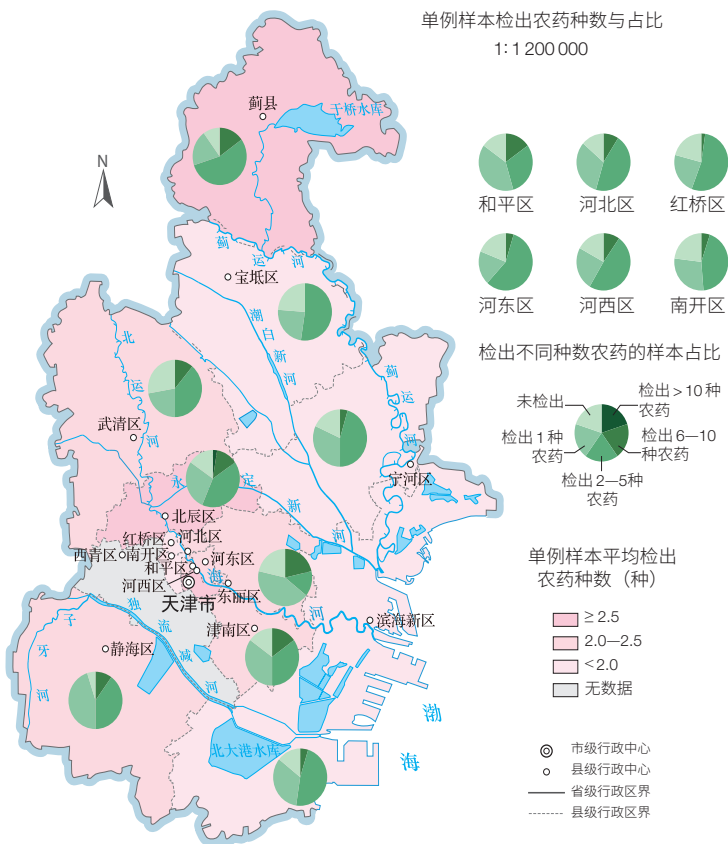
图6 天津市水果蔬菜样品检出农药品种与占比 (%)
