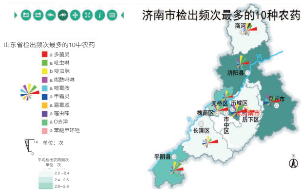
图 18 济南市检出频次最多的10种农药分布
