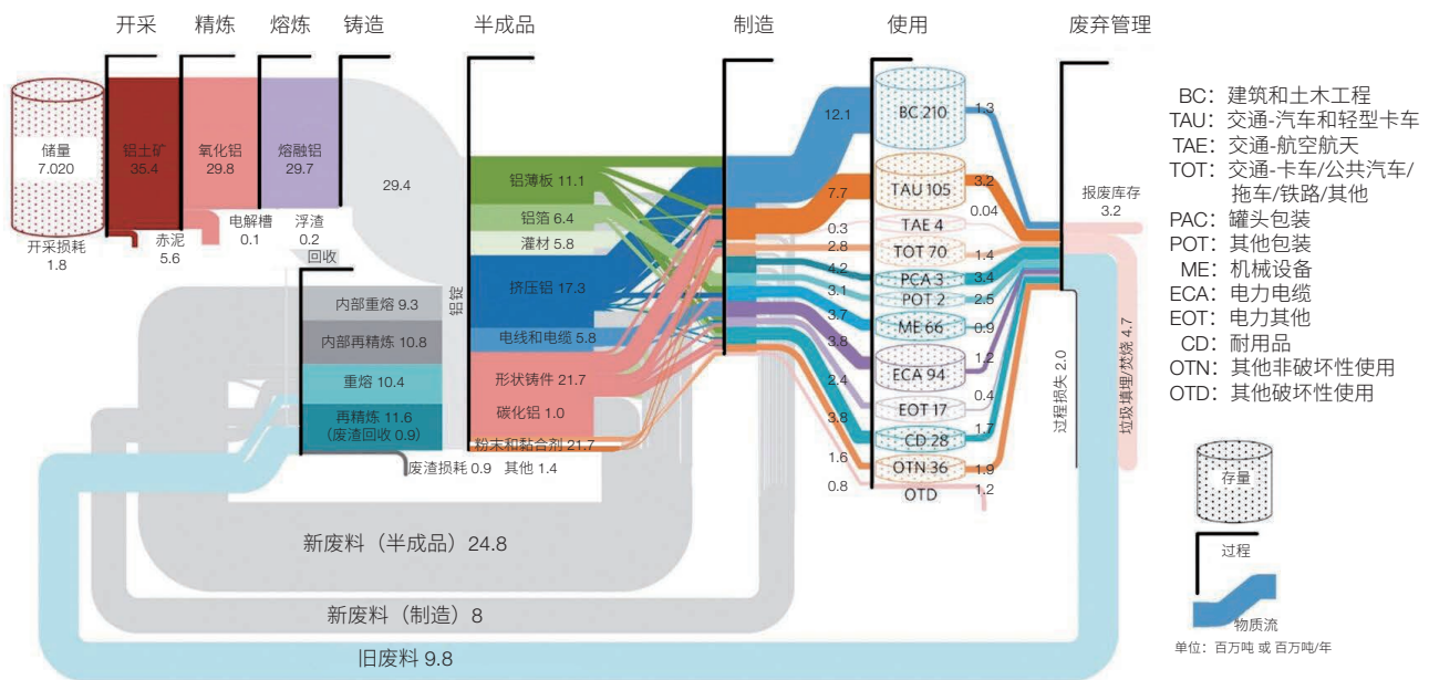
图3 2009年全球铝元素循环图（转译自文献[32]）
