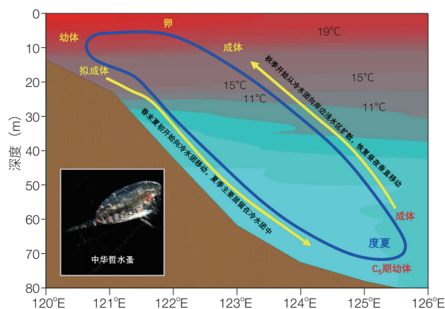
图1 中华哲水蚤度夏机制
