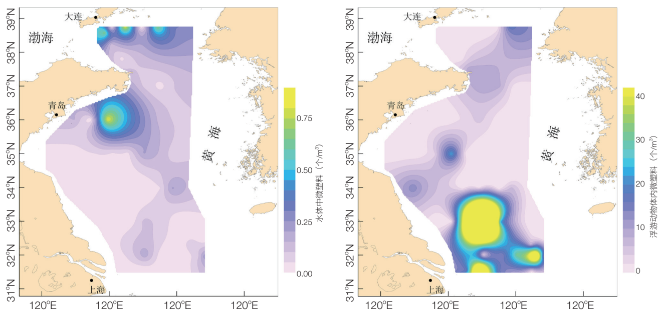
图8 黄海海水与浮游动物体内微塑料分布
