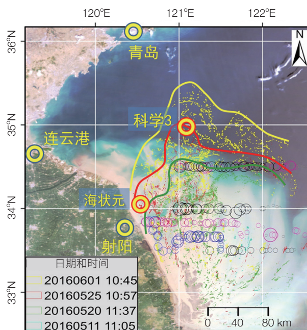
图6 黄海绿潮漂移路径追踪
