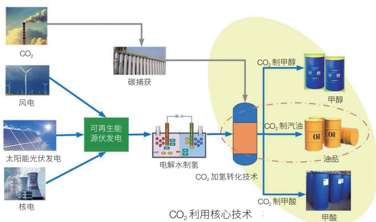
图 4 零碳能源耦合二氧化碳的转化利用路线图
