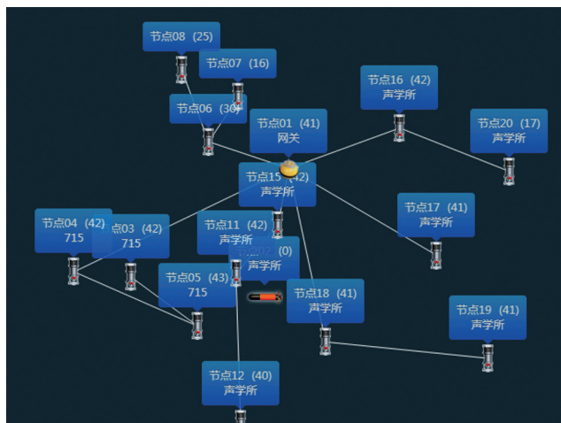
图3 水声通信海上试验网络拓扑结构图(连线表示通信链路)
