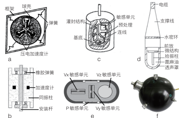
图 8 矢量水听器
