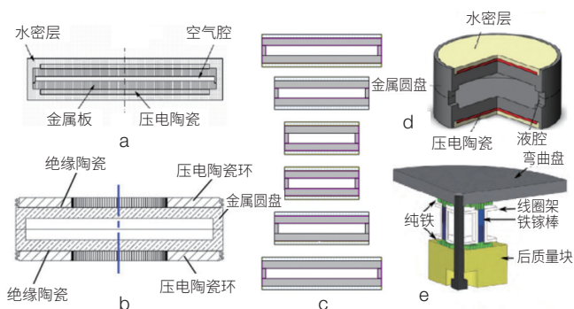
图2 弯曲圆盘低频换能器的新设计
