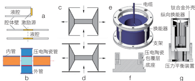
图 7 深水换能器
