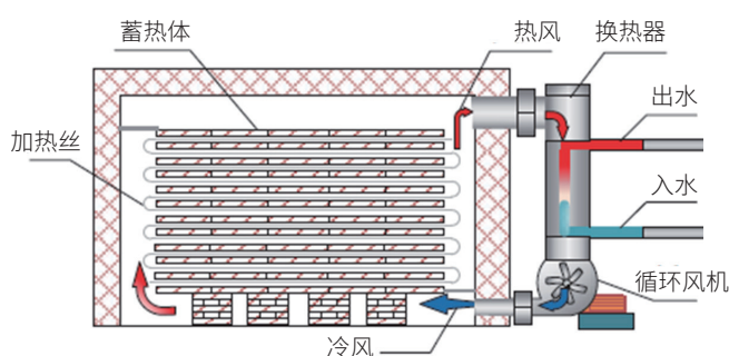
图 4 大规模高压电制热蓄热供暖系统结构简图 [22]
