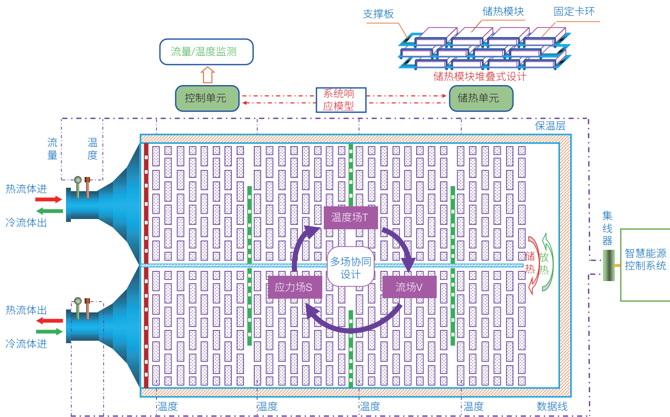
图7 可移动式烟气余热储热供暖装置结构简图 [26,27]
