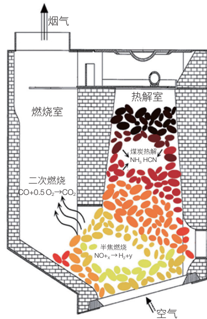
图2 解耦炉结构示意图 [17]
