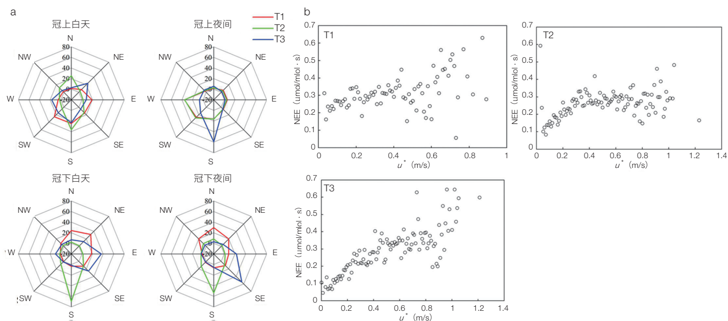
图3 风格局及其与生态系统碳净交换的关系
