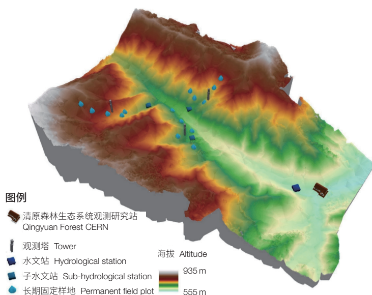
图 1 科尔塔群所在流域的地形图 [5]
