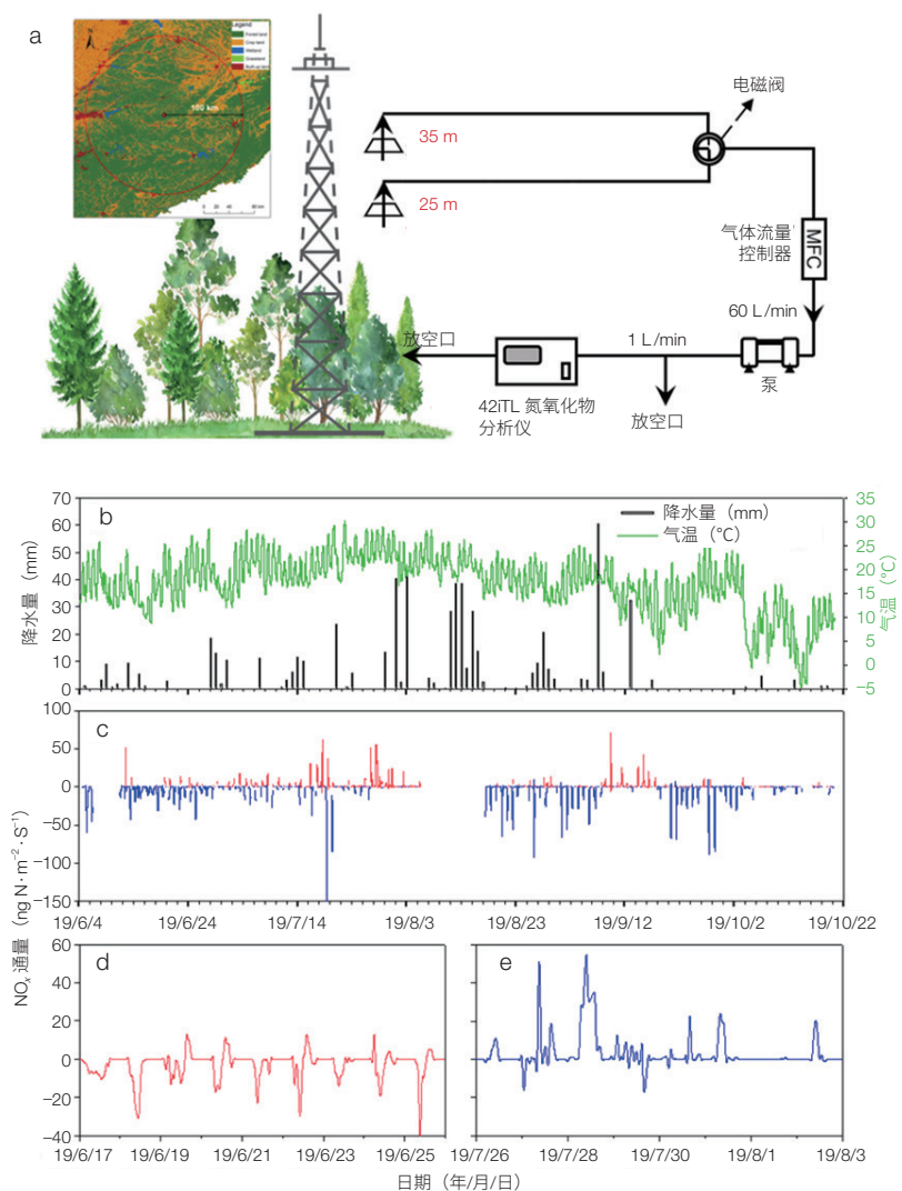
图4 典型次生林林冠以上氮氧化物( \text{NO}_x )通量观测结果
